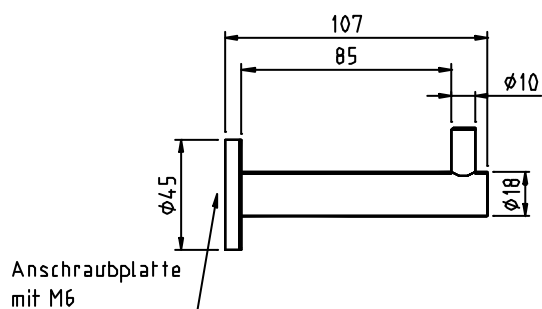
1328.100 Wandhaken Edelstahl Anschraubplatte siehe Seite 7.1
