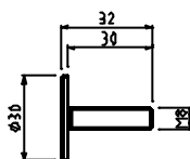
2018.30 Edelstahl-Schraube, Stellfuß oder Abschluss, eignet sich zur Glasplattenverklebung
