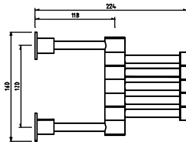
4123 Wandgarderobe in Edelstahl mit 5 schwenkbaren Haken.
