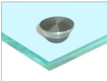
1112 Mini-Puffer Edelstahl/Gummi Ø20 x 10 mm zum Verkleben auf Glas oder als Auflage
