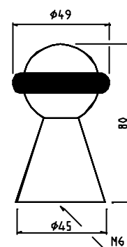
1105 Türstopper in Alu zum Anschrauben
