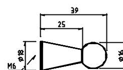
1196G Wandhaken mit Gummikugel
