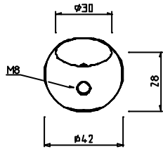
2010... Kugelverbindung 1 - 4 Anschlüsse
